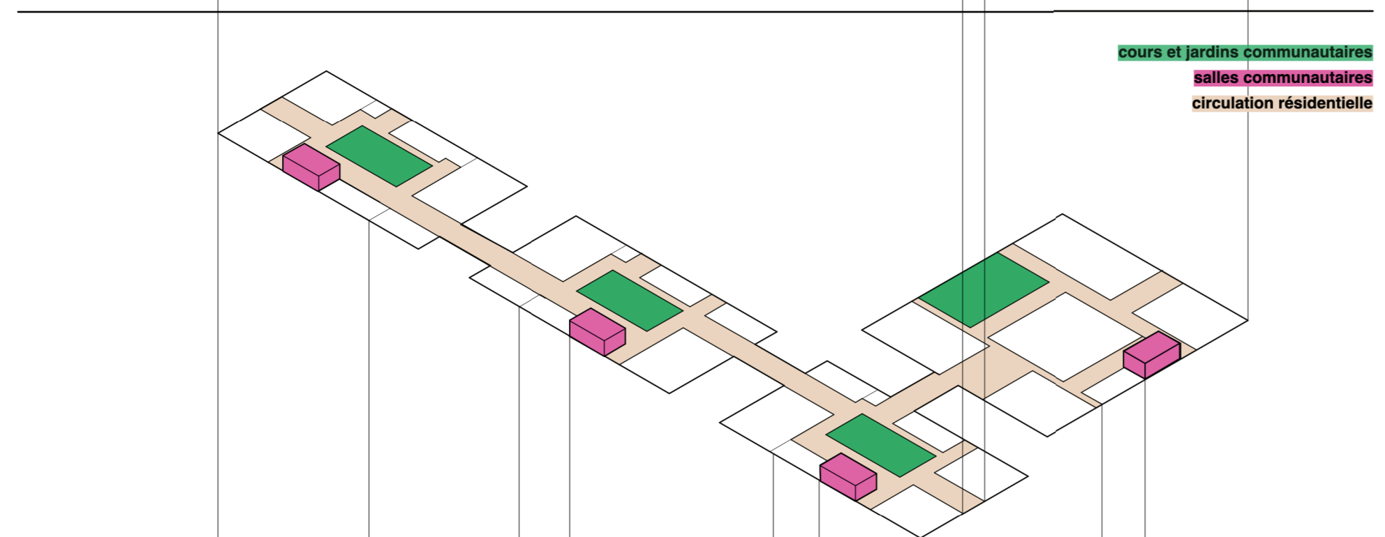
NIVEAU COLLECTIF [+2]
